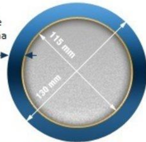
Esquema de una sección transversal del cuerpo de la HP 130.
